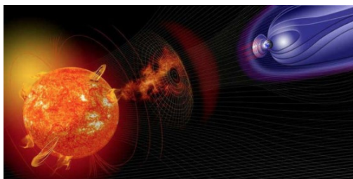
Les éjections coronales saturent les espaces interplanétaires
